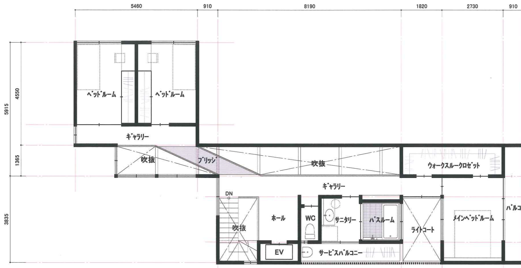
2階平面図
