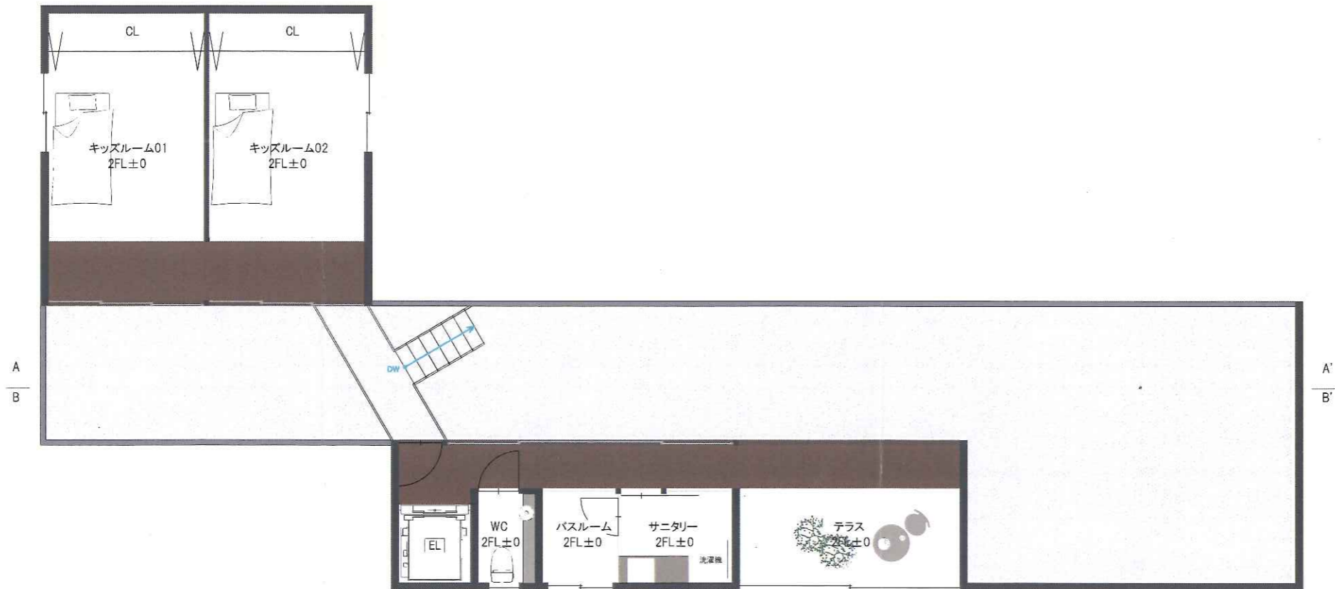
2F平面図
